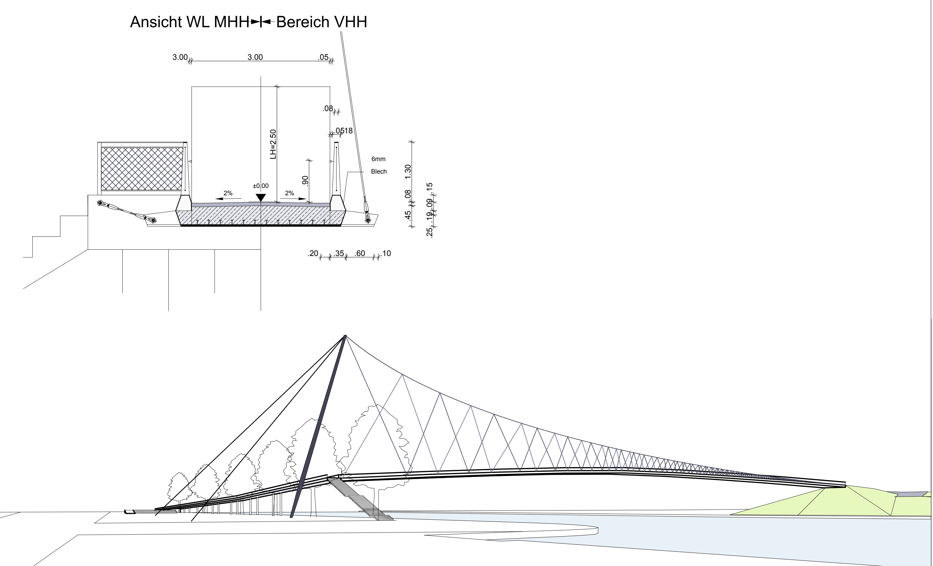
Regelquerschnitt M 1:50
