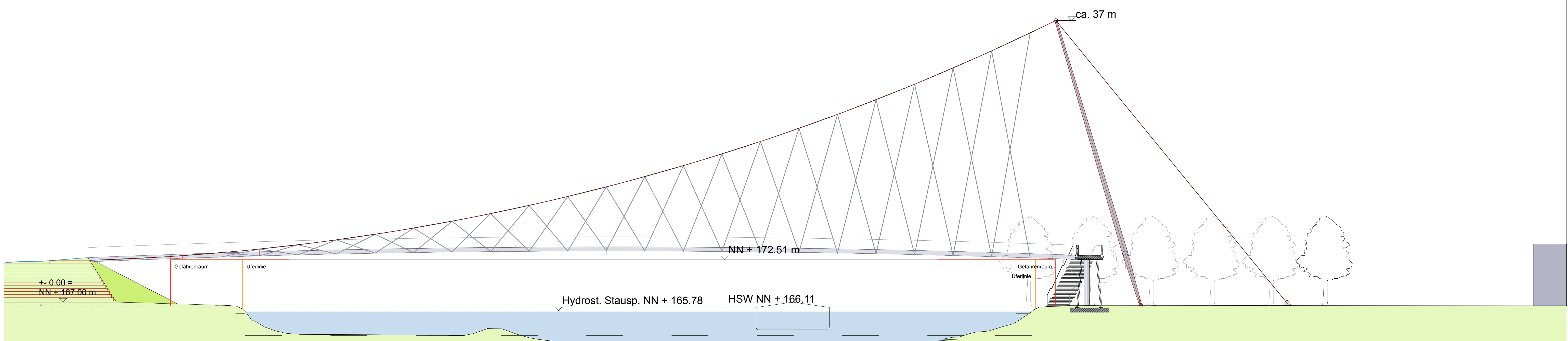
Ansicht M 1:250
