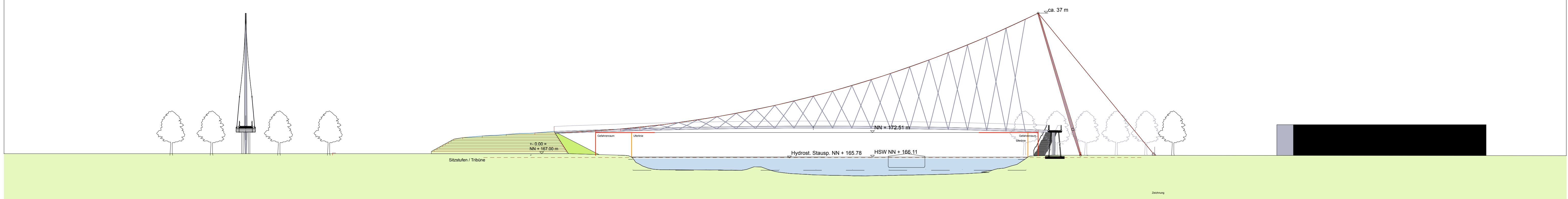
Querschnitt M 1:500
