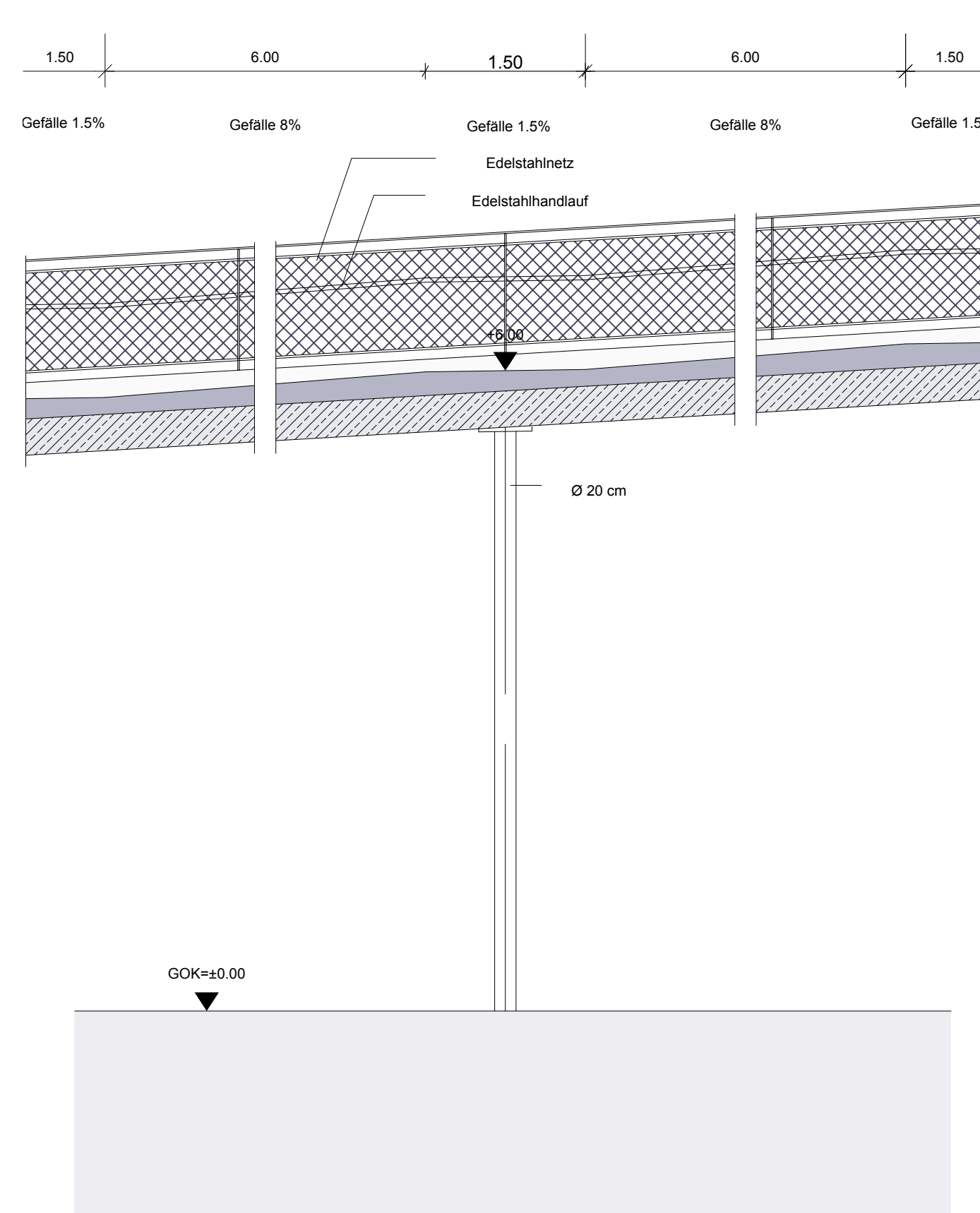
Rampenlängsschnitt M 1:50
